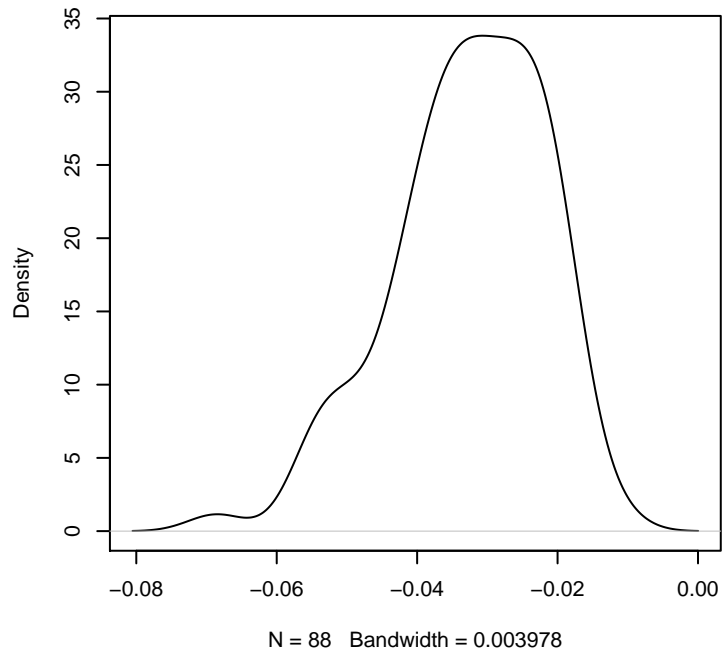
b) Density of (h2FMM-h2Old)
